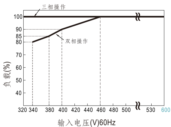
■ 输出减额 VS 输入电压
